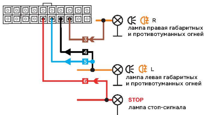
1. Схема подключения для односторонней лампы реализует функцию габаритных и противотуманных огней.
