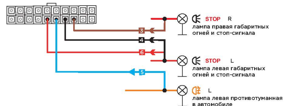
2. Схема подключения для односторонней лампы реализует функцию габаритных огней и стоп-сигнала.
